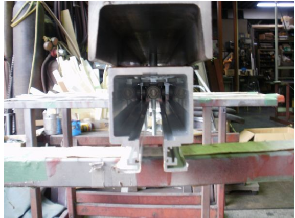
写真 - 2 引張りテスト前試験体セット
